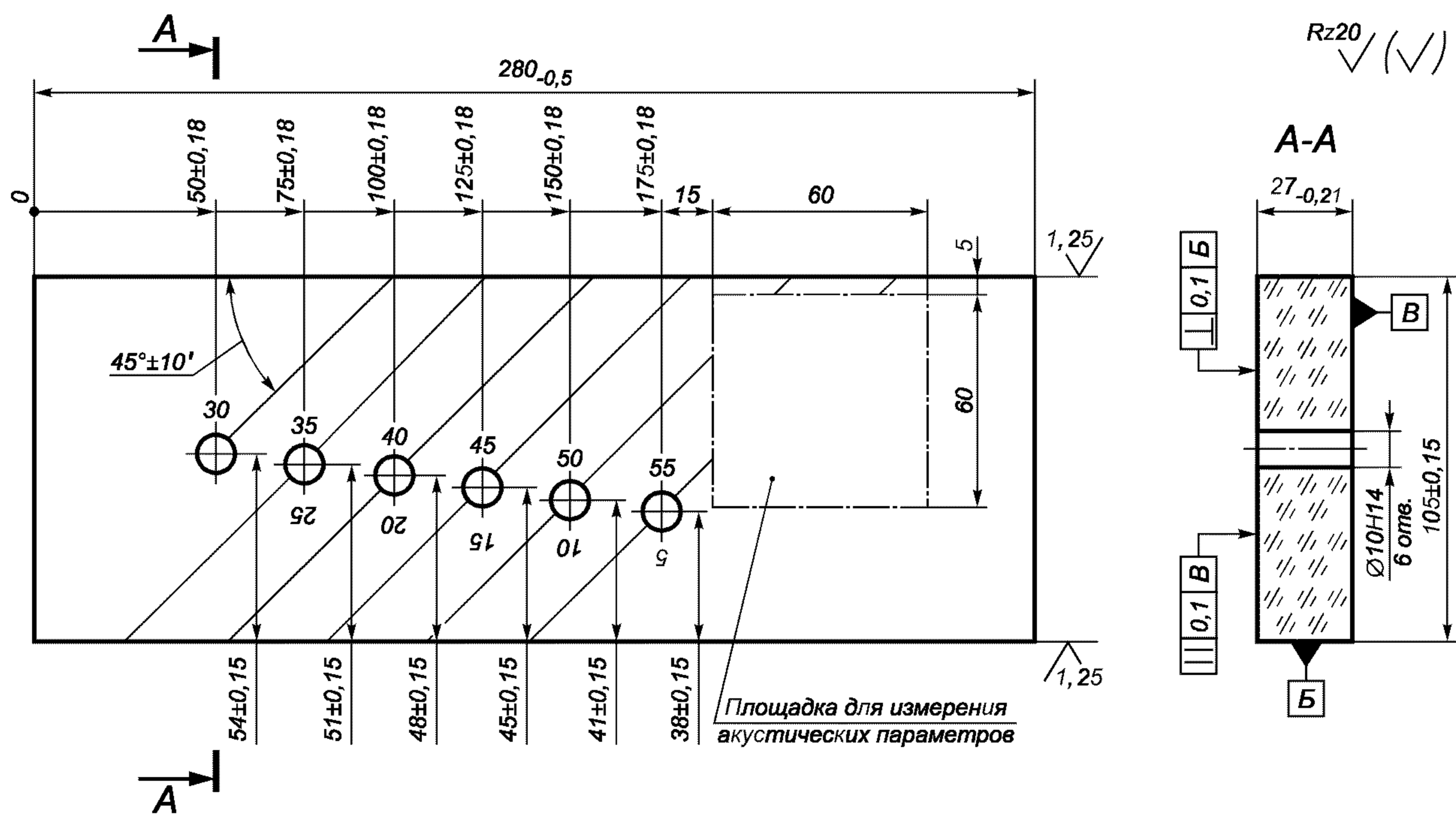
Рисунок 2 — Стандартный образец СО-1Р
